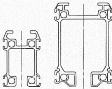
图2 压铸铝合金型轨截面
