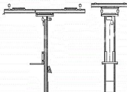
图7 堆垛型式
