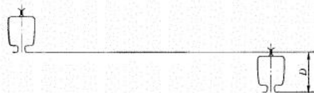
图 9 起重机两轨道在同一截面处的高度差
