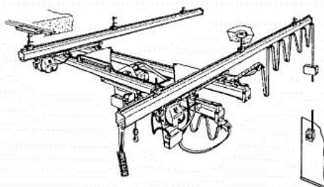
图5 双梁悬挂型式
