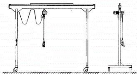
图6 门架型式
